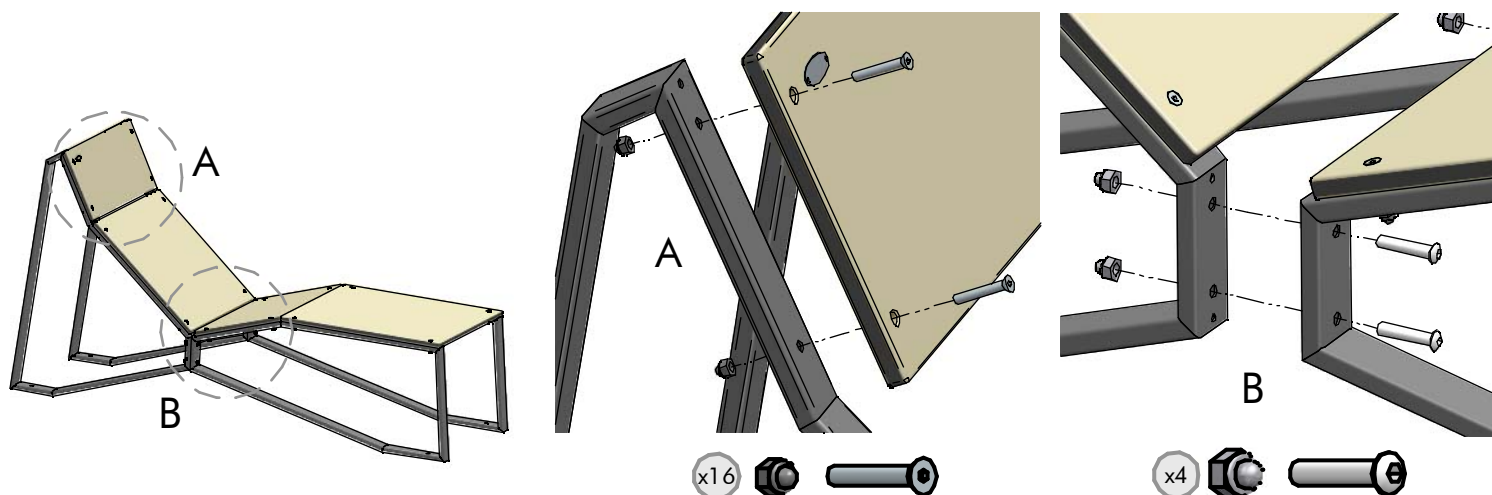
DETALLE DE MONTAJE/ ASSEMBLY DETAIL/ INSTRUCTION DE MONTAGE
