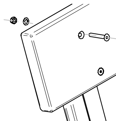
DETALLE DE MONTAJE ASSEMBLY DETAIL INSTRUCTION DE MONTAGE
